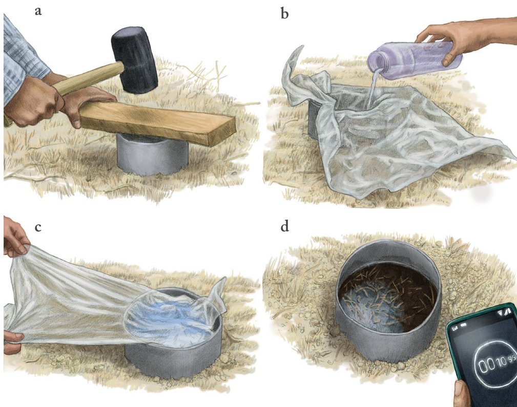
Figura 6. Para medir la infiltración, BIOCOMUNI cronometra el tiempo en que el suelo absorbe una pulgada de agua.
