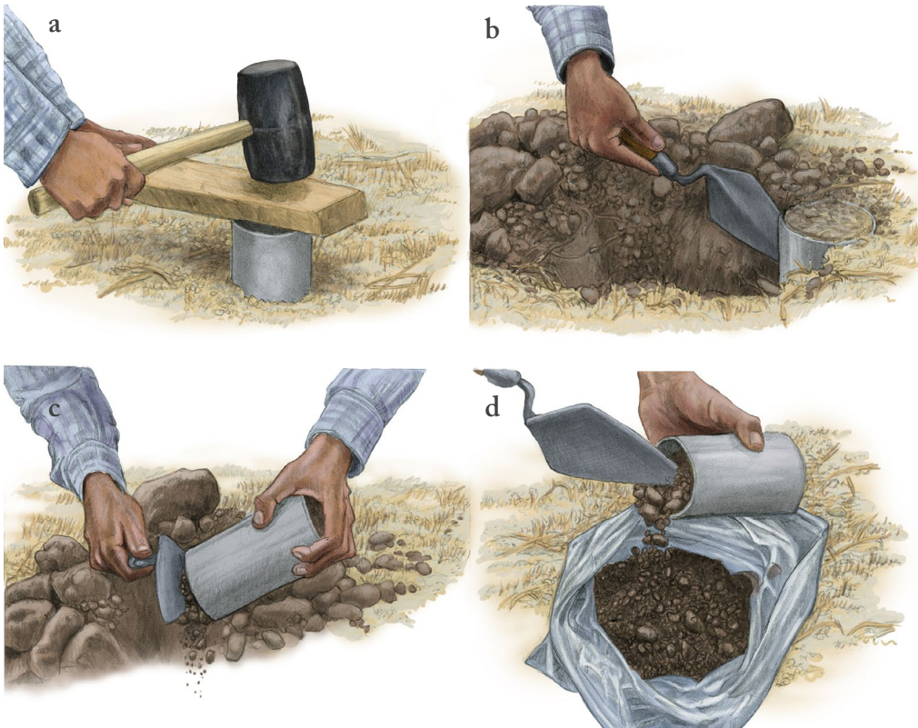
Figura 7. Para medir la densidad aparente, la brigada entierra el tubo de acero para coleccionar una muestra de suelo que llevará a la comunidad para pesar, secar y volver a pesar.
